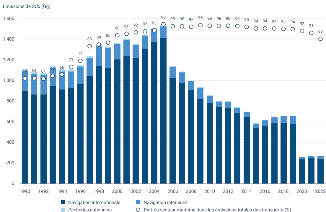
Figure 5 Émissions de SOx du secteur maritime (Gg) et leur part dans les émissions totales du secteur des transports (%) entre 1990 et 2022 dans l'UE-27
