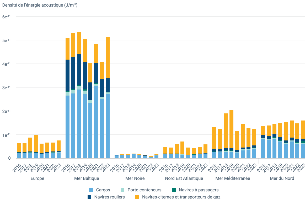
Figure 9 Densité d'énergie sonore du bruit sous-marin rayonné à 63 Hz en Europe et dans les mers régionales de 2016 à 2023
