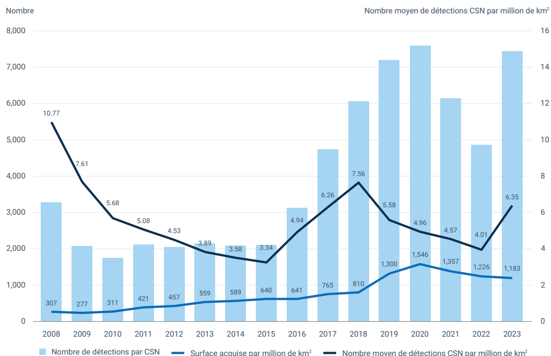
Figure 7 Évolution du nombre annuel de potentiels déversements détectés par CleanSeaNet et du nombre moyen de potentiels déversements par million de km 2
