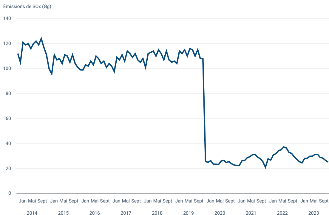
Figure 4 Émissions de SOx pour l'UE, 2014-2023
