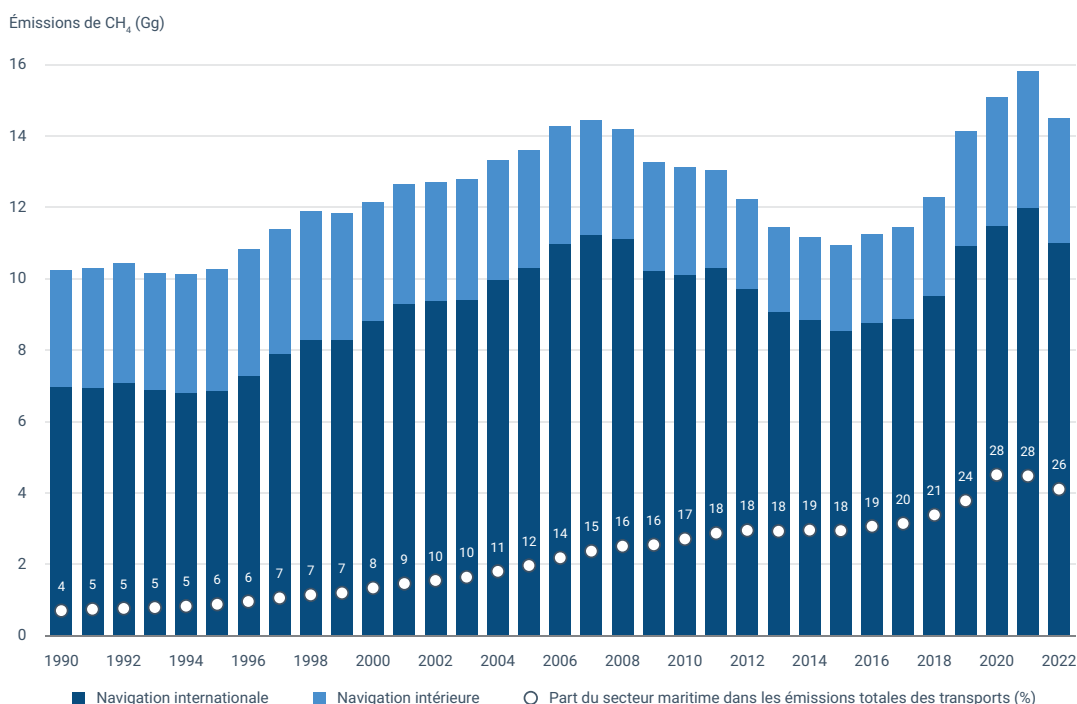
Figure 3 Les émissions de CH 4 du secteur maritime (Gg) et leur part dans les émissions totales des transports (en%) entre 1990 et 2022 dans l'UE-27
