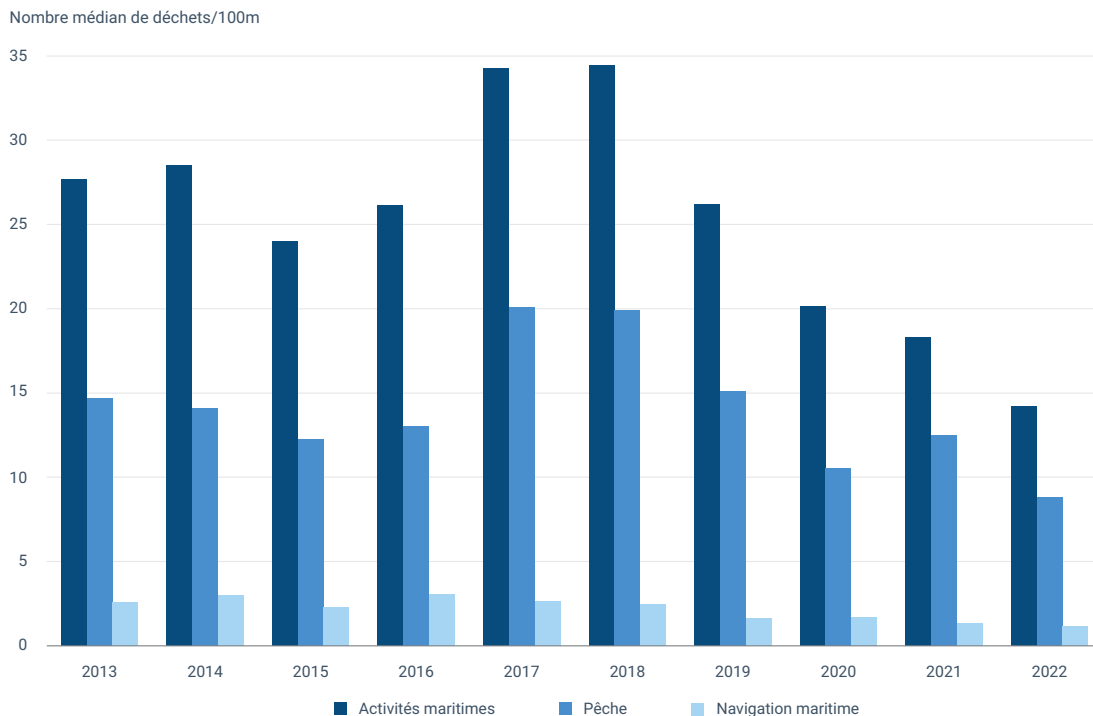
Figure 12 Distribution temporelle des déchets susceptibles de provenir de l'ensemble des activités maritimes, des transports maritimes, de la pêche et de la mariculture, dans les mers régionales européennes
