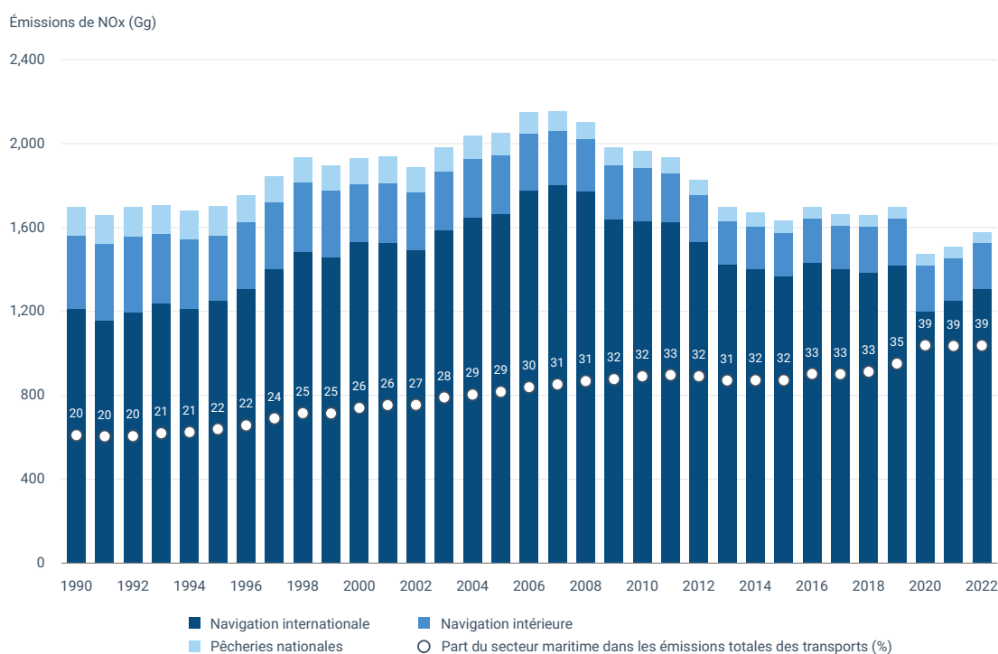
Figure 6 Les émissions de NOx du secteur maritime (Gg) et leur part dans les émissions totales des transports (%) entre 1990 et 2022 dans l'EU-27
