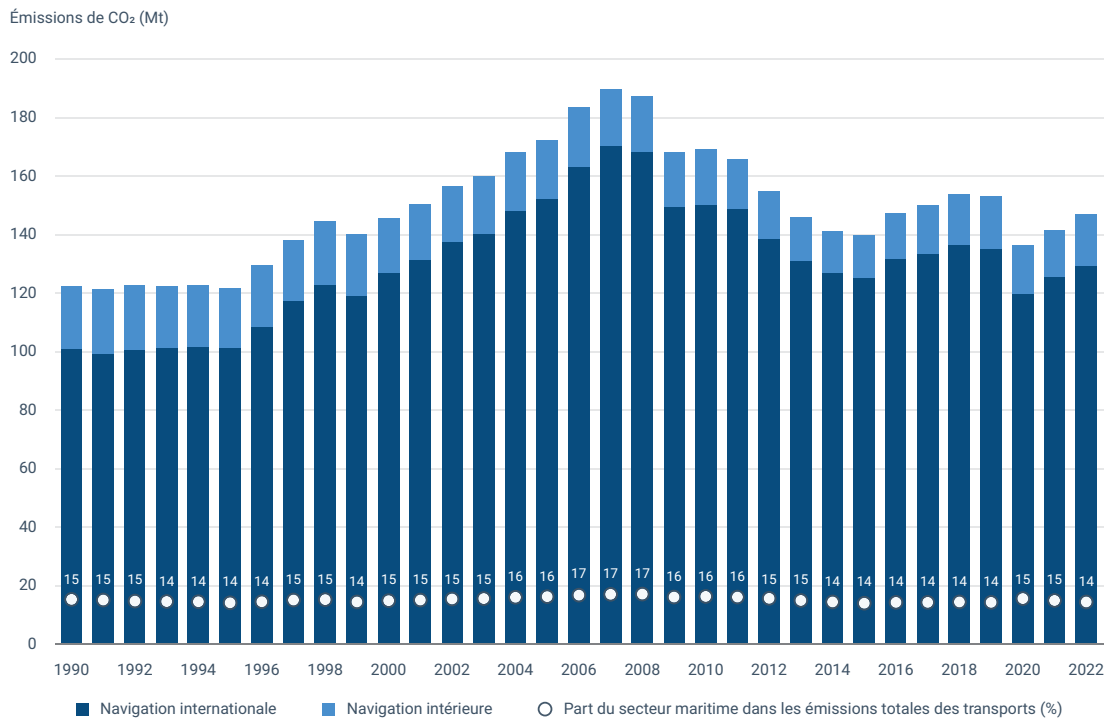
Figure 1 Les émissions de CO 2 du secteur maritime (Mt) et leur part dans les émissions totales des transports (%) entre 1990 et 2022 dans l'EU-27
