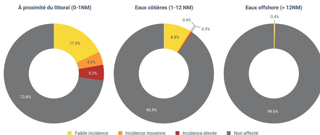
Figure 10 Pourcentage de fonds marins physiquement perturbés dans les eaux proches du rivage (0-1NM), les eaux côtières (1-12NM) et les eaux du large (>12NM) dans les mers régionales
