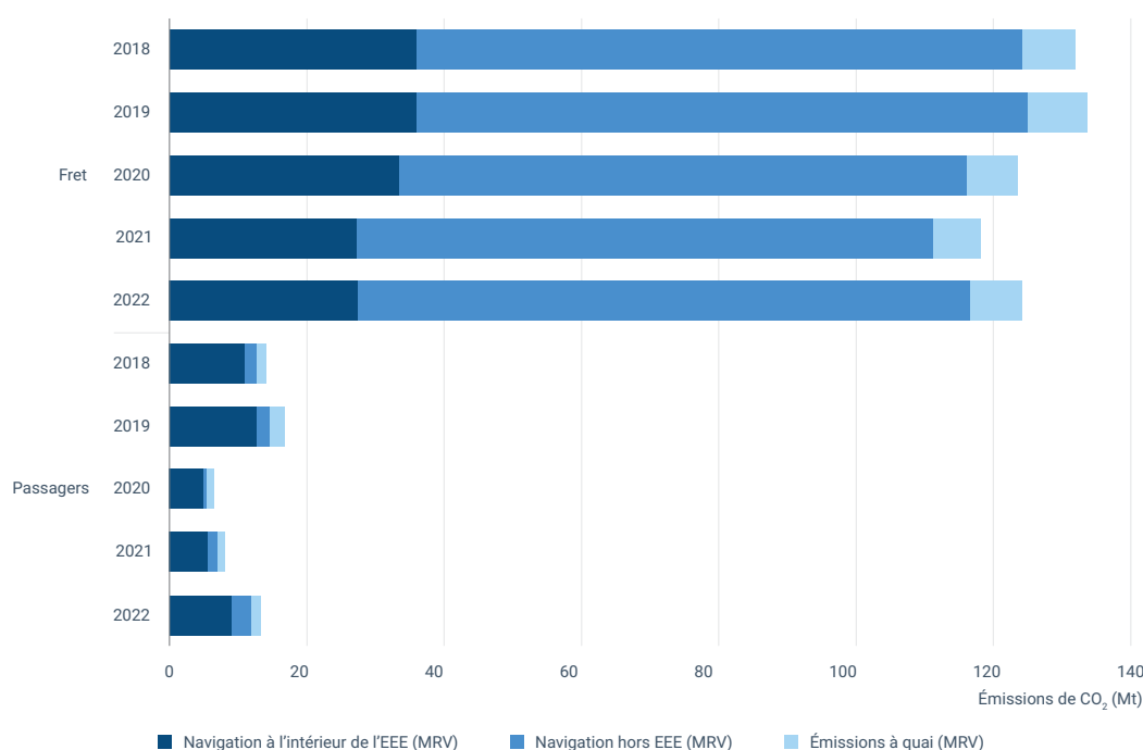
Figure 2 Répartition des émissions de CO 2 des navires de transport de marchandises et de passagers entre 2018 et 2022 dans l'Espace économique européen
